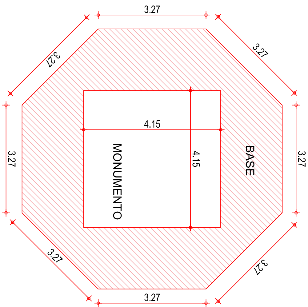
DETALHE 01
