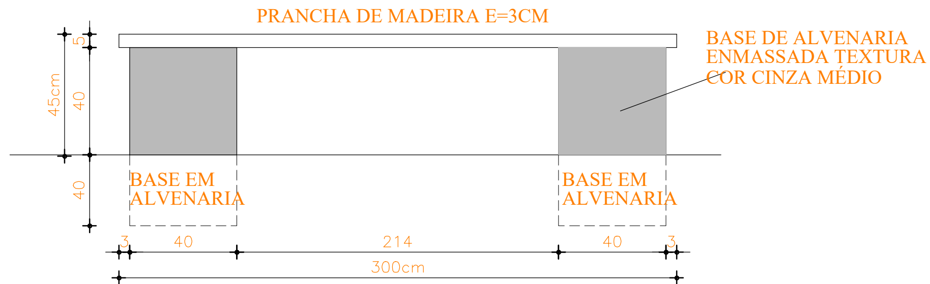
2 VISTA FRONTAL DO BANCO ESCALA: 1 / 30
