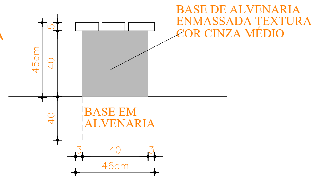
3 VISTA LATERAL DO BANCO ESCALA: 1 / 30
