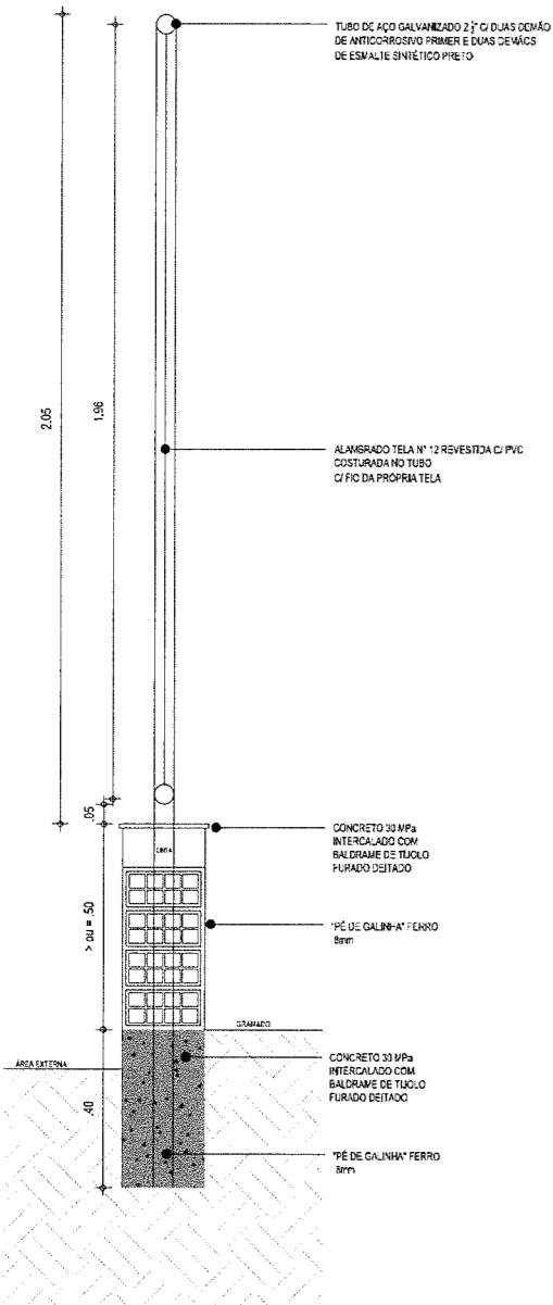
05 | CORTE/DET. MURETA ESC.: 1/20
