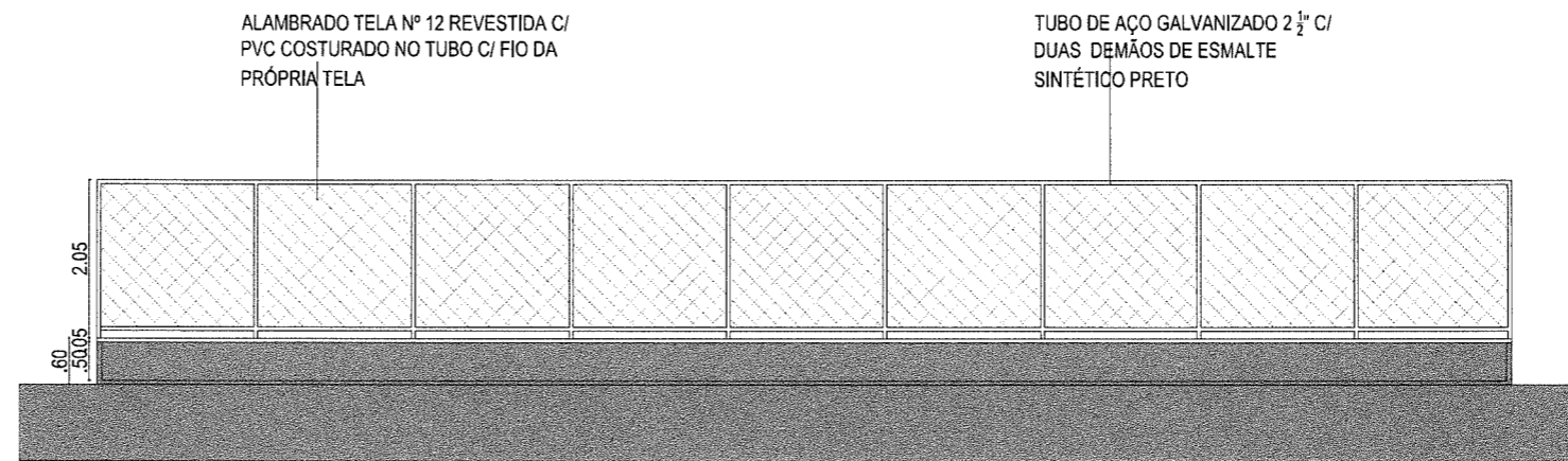
03 | FACHADA F1 ESC.: 1/100
