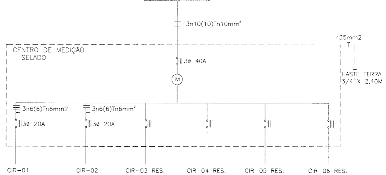
ESQUEMA TRIFILAR GERAL COELCE 380/220V
