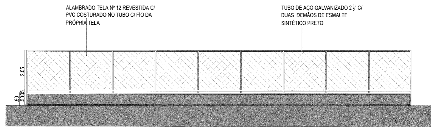
03 FACHADA F1 ESC.: 1/100
