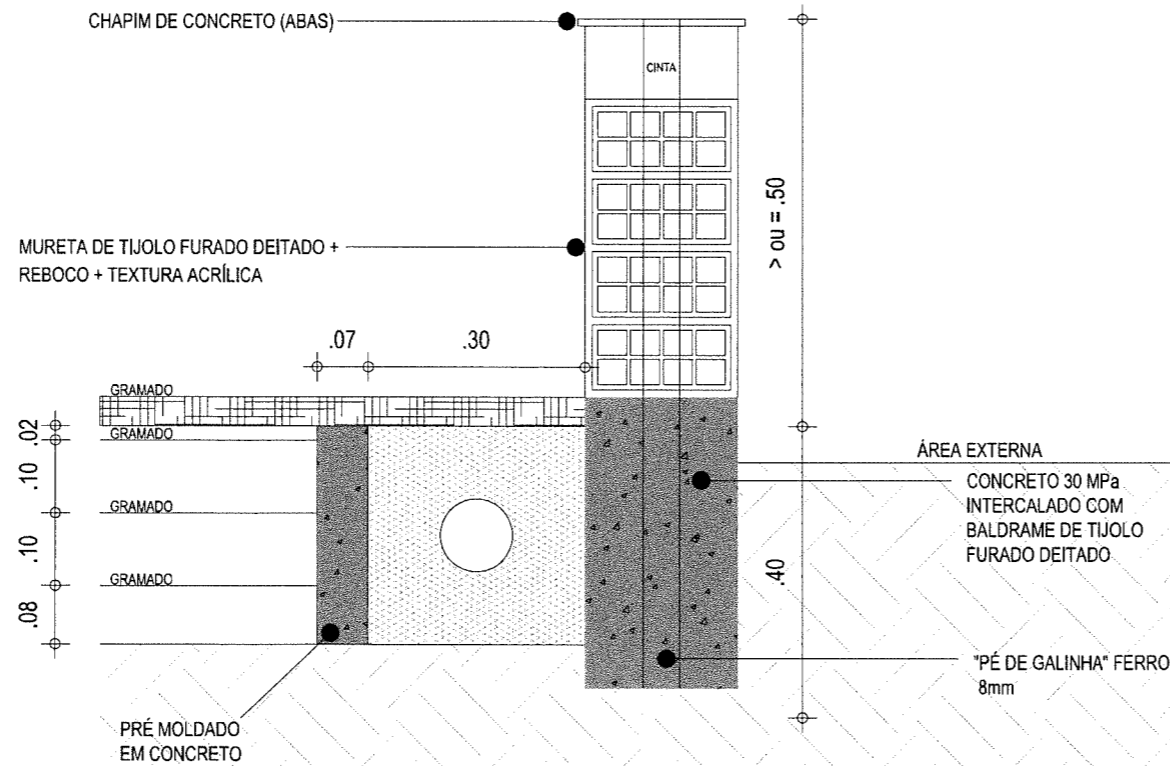
06 | CORTE/DET. INSTALAÇÕES ESC.: 1/10
