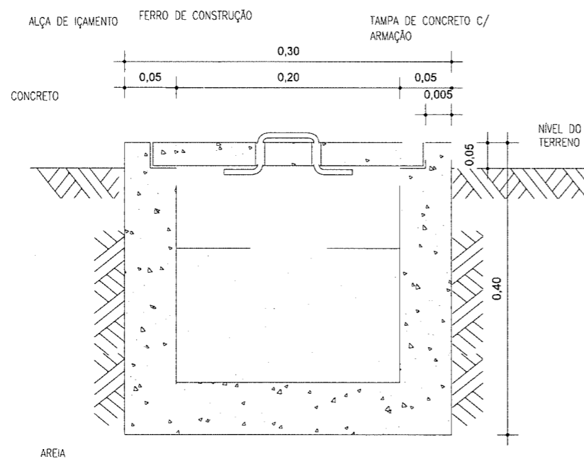
DET. CAIXA DE CONCRETO PARA POSTE DE ILUMINAÇÃO
