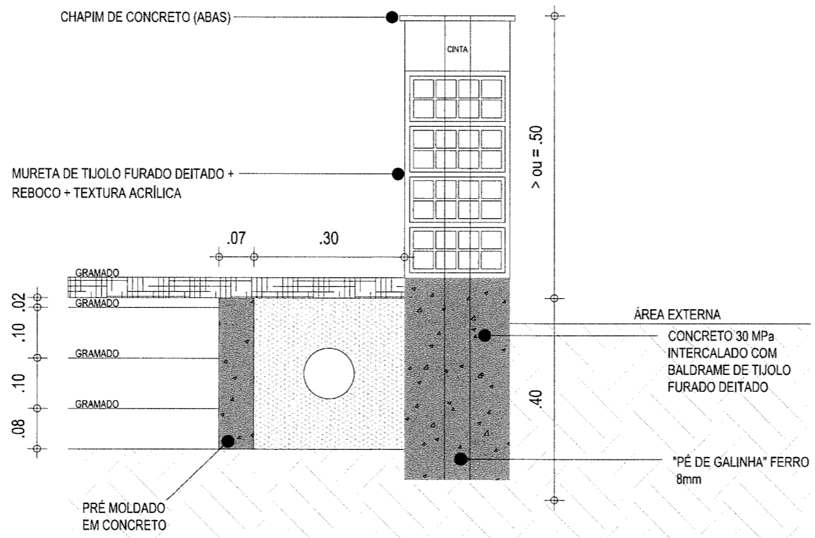
06 CORTE/DET. INSTALAÇÕES ESC.: 1/10
