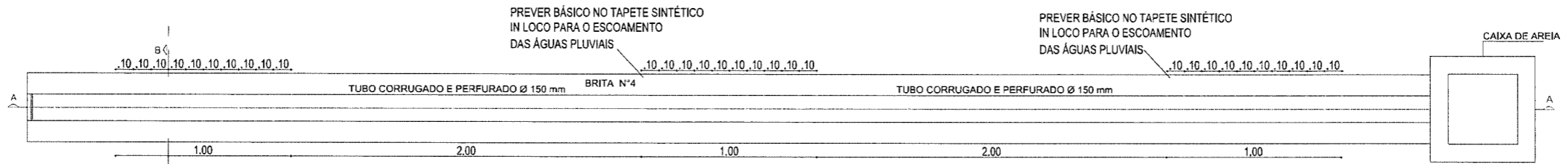
PLANTA BAIXA - VALA DE INFILTRAÇÃO
