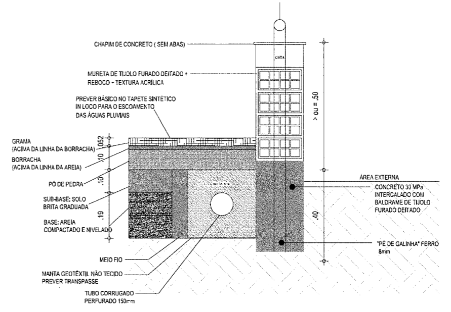
CORTE B:B
