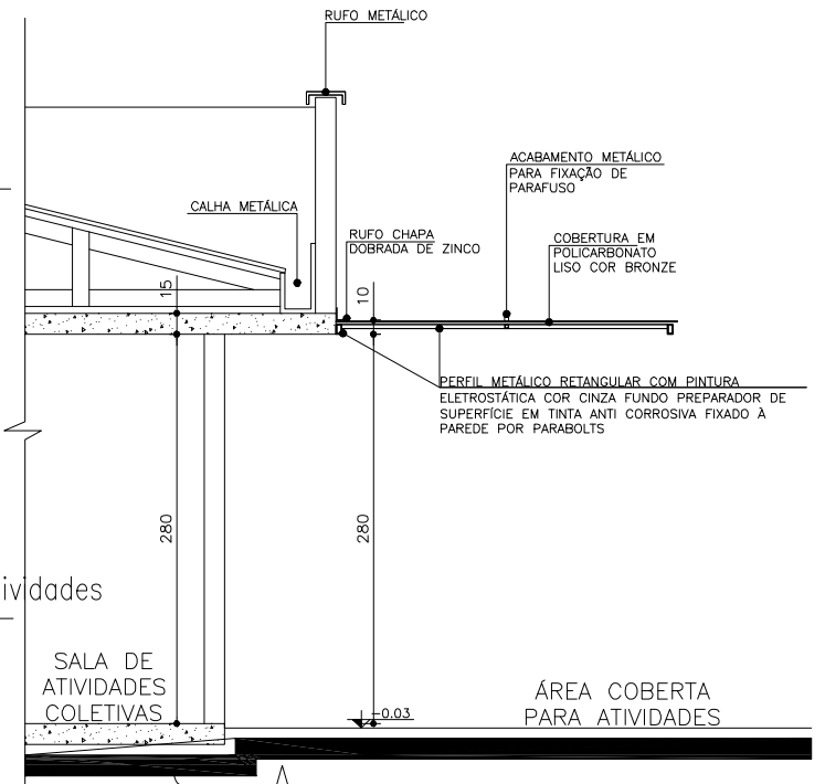
06 S AA'-Marquise Sala de Atividades
